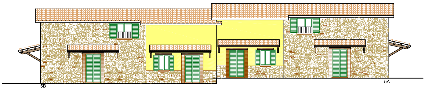
PROSPETTO OVEST
