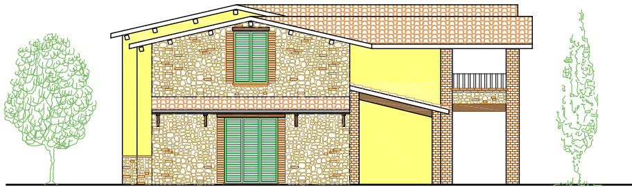
PROSPETTO NORD
