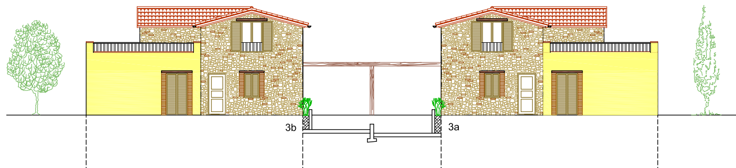
PROSPETTO OVEST
